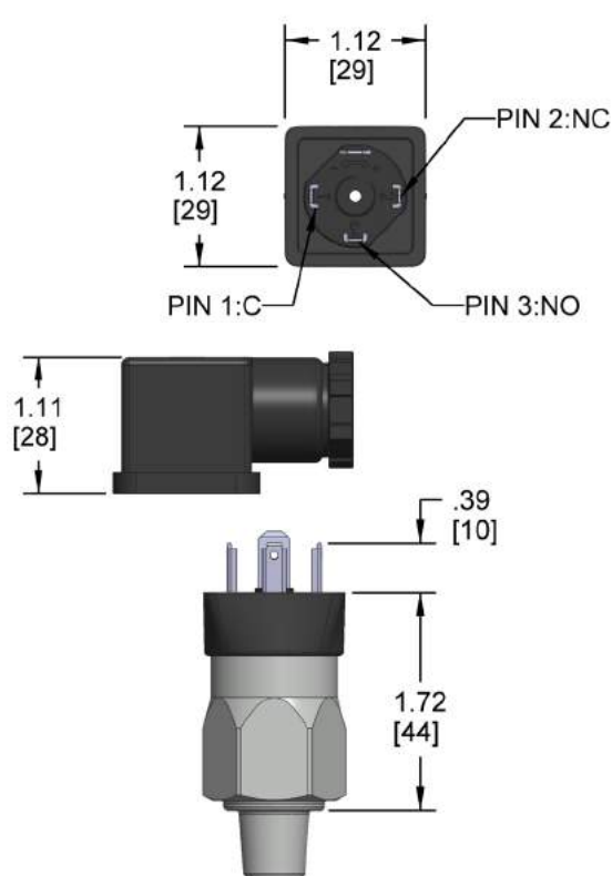
200H DIN EN 175301-803 Form A
