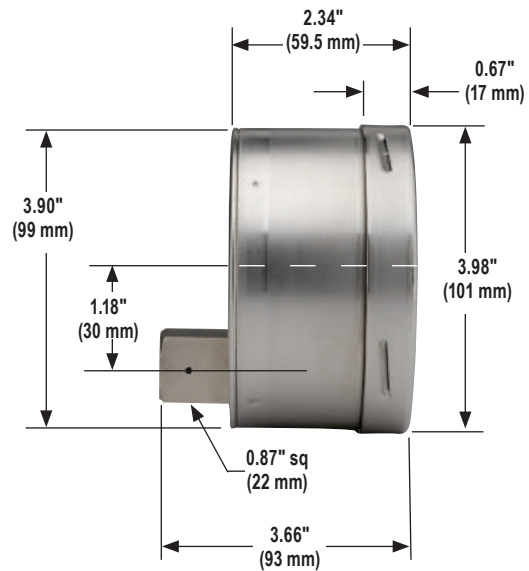
40-412
