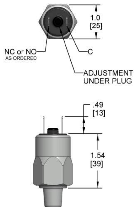
200H DIN EN 175301-803 Form A
